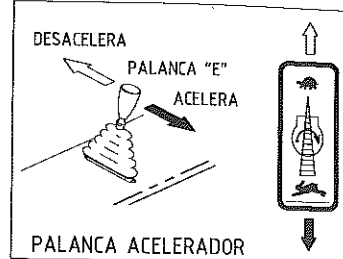
PALANCA ACELERADOR
