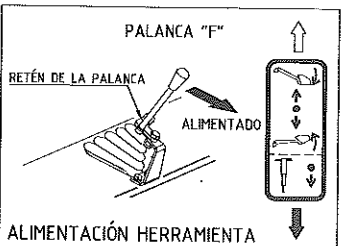
ALIMENTACIÓN HERRAMIENTA
