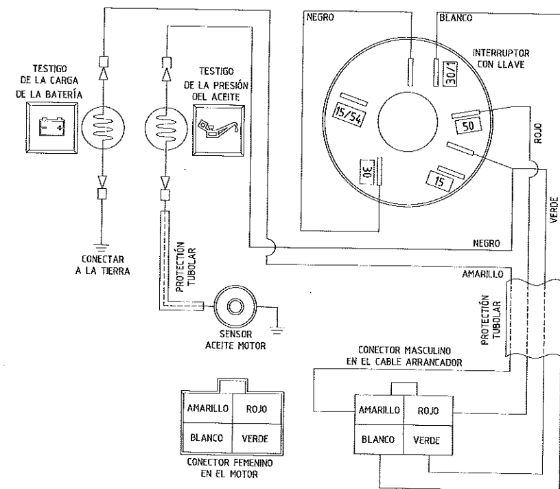
INTERRUPTOR DE ARRANQUE
