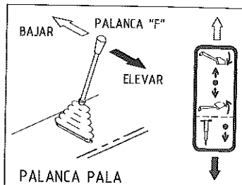
PALANCA PALA
