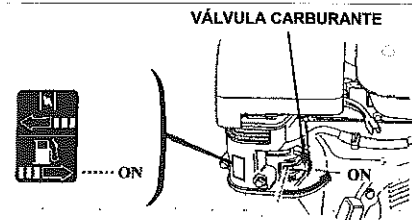
VÁLVULA CARBURANTE
