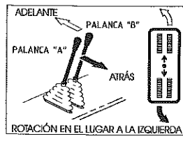
ROTACIÓN EN EL LUGAR A LA IZQUIERDA
